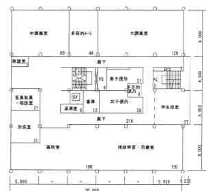
3階平面図 S=1/400
