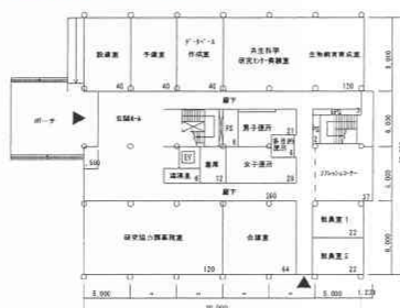
1階平面図 S=1/400
